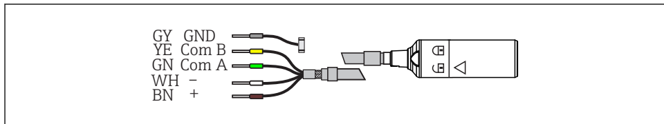
3 Измерительный кабель CYK10 или CYK20
