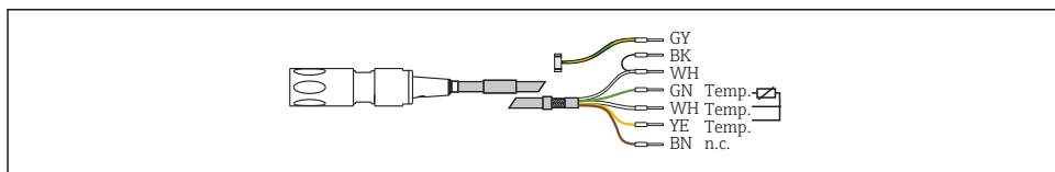
4 Измерительный кабель CPK9
